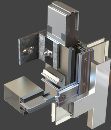
Classic Cam Giydirme Cephe Sistemi
